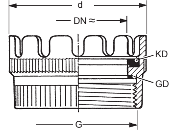
Деталь TW-K
